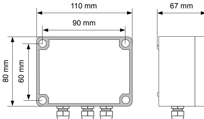
Rys. 4.1. Wymiary montażowe
