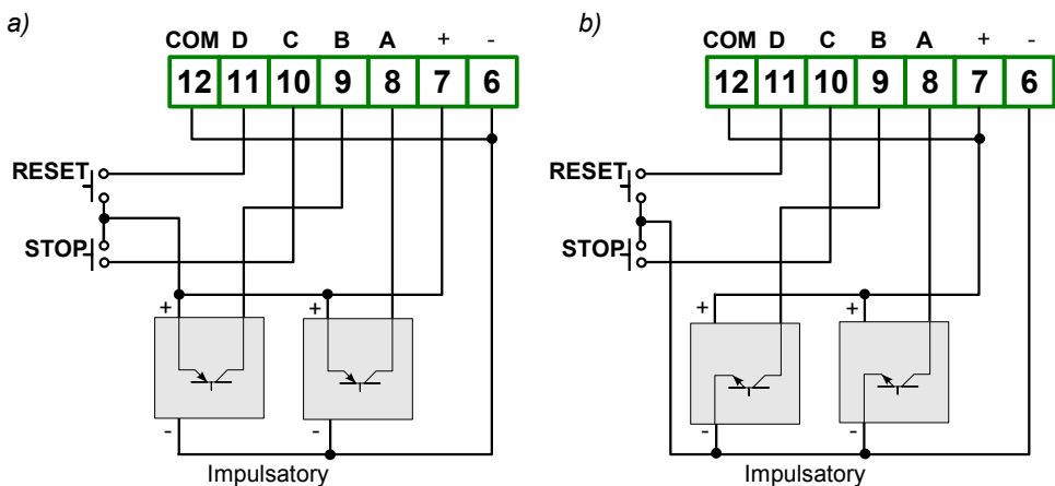
Rys. 4.8. Przykład podłączenia czujnika obrotowo-impulsowego: a) ze wspólną masą, b) ze wspólnym plusem
