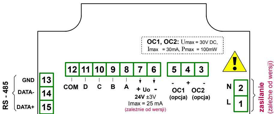
Rys. 4.4. Opis wyprowadzeń dla wersji z wyjściem OC
