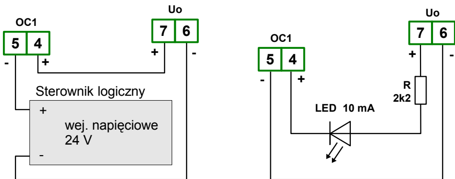
Rys. 4.7. Przykładowe podłączenia wyjścia typu OC
