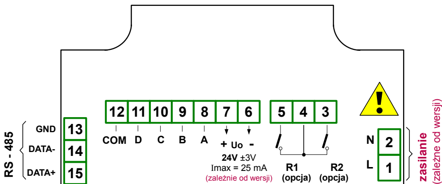
Rys. 4.3. Opis wyprowadzeń dla wersji z wyjściem przekaźnikowym
