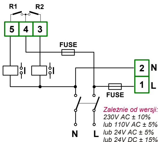
Rys. 4.5. Podłączenie zasilania oraz przełączników sterujących obciążeniami
