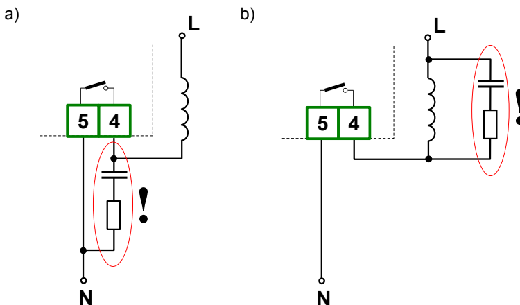
Rys. 4.6. Przykłady równoległego podłączenia obwodu tłumiącego: a) do styków przełącznika; b) do obciążenia indukcyjnego
